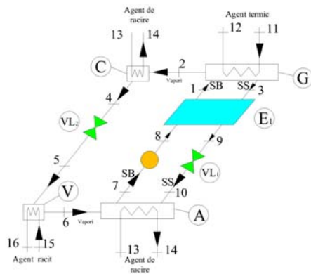
Fig. 6. EES schematic
